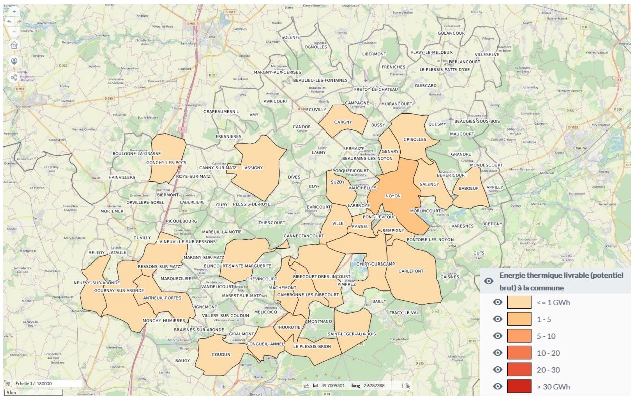
Figure 35 : Gisement brut total d'énergie thermique livrable sur les filières eaux usées, blanchisseries et data centers – Source OPPORTUNITE BURGEAP
