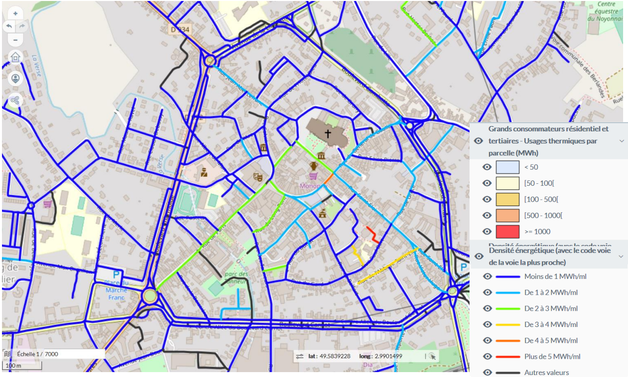
Figure 42 : Potentiel de développement réseaux de chaleur à Noyon centre – Source OPPORTUNITEE BURGEAP
