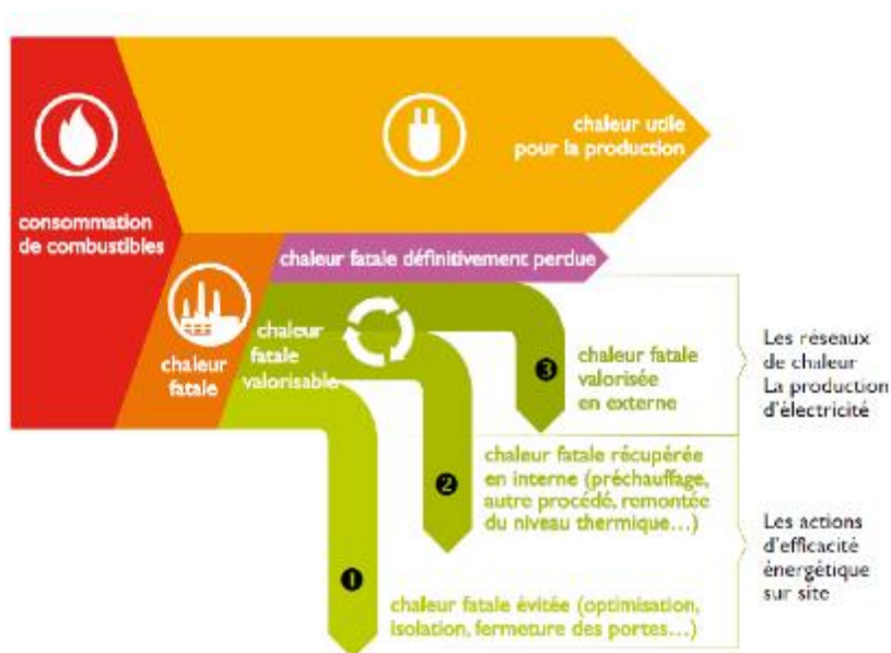
Figure 34 : La récupération de chaleur fatale – Source ADEME, juillet 2015
