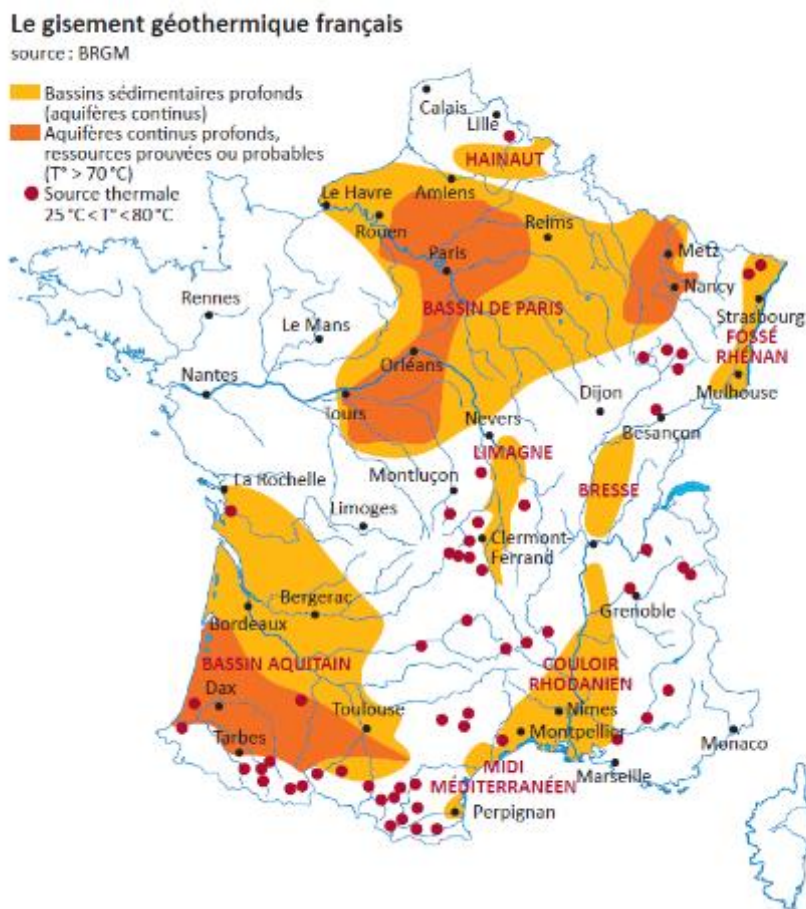
Figure 25 : Cartographie du gisement géothermique Français – Source BRGM
