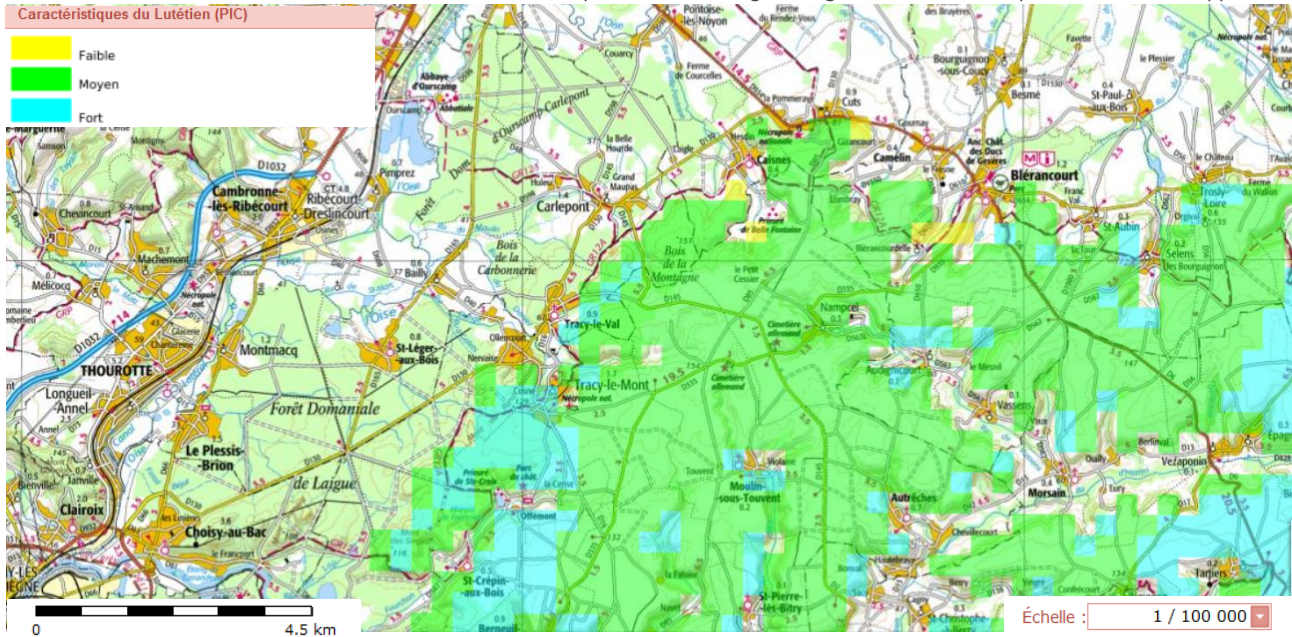
Figure 29 : Gisement géothermique sur aquifère profond (Lutétien) – Source géothermie-perspectives
