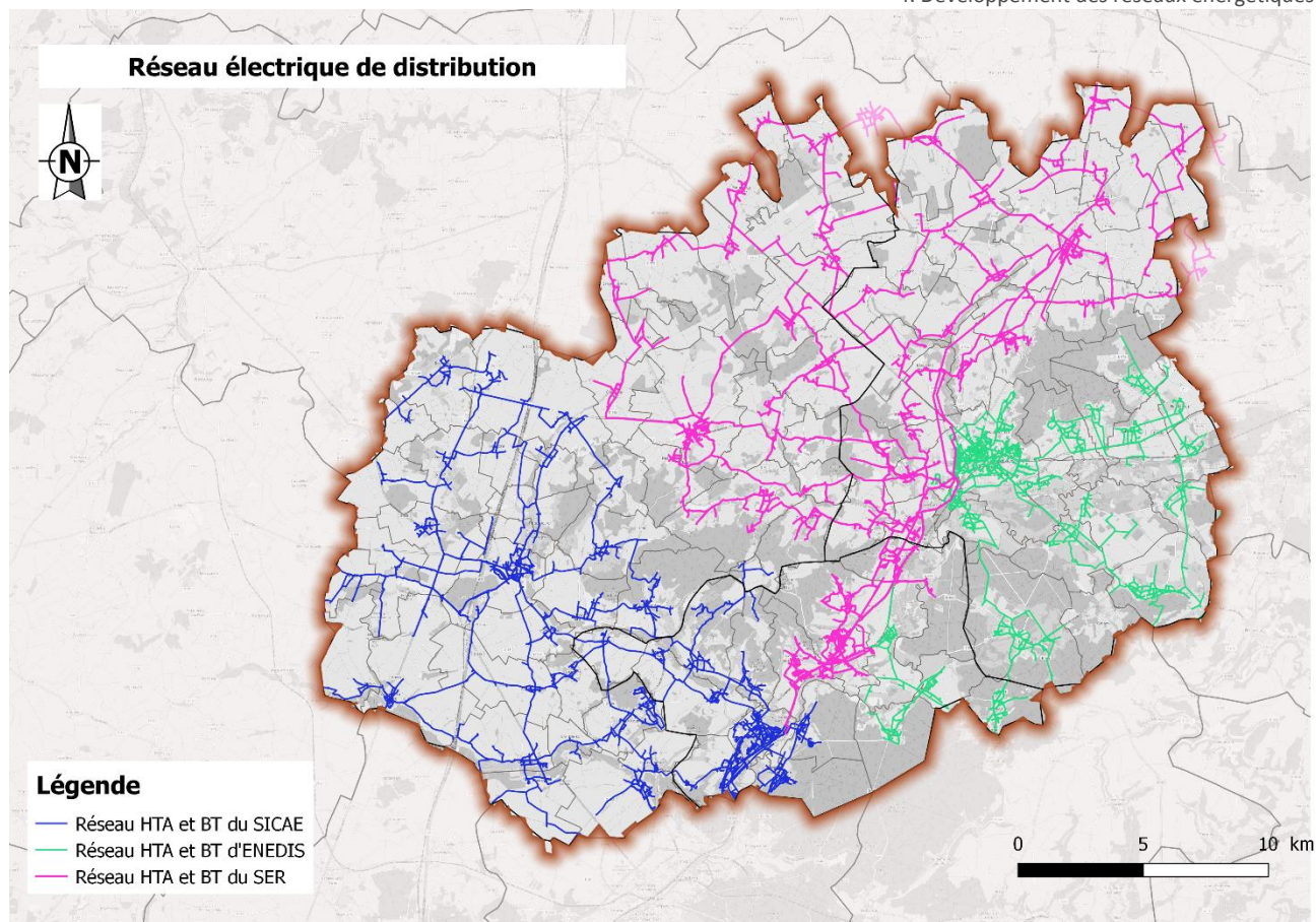
Figure 41 : Réseau de distribution d'électricité géré par ENEDIS et les deux ELD du territoire – Source ENEDIS, SICAE, SER
