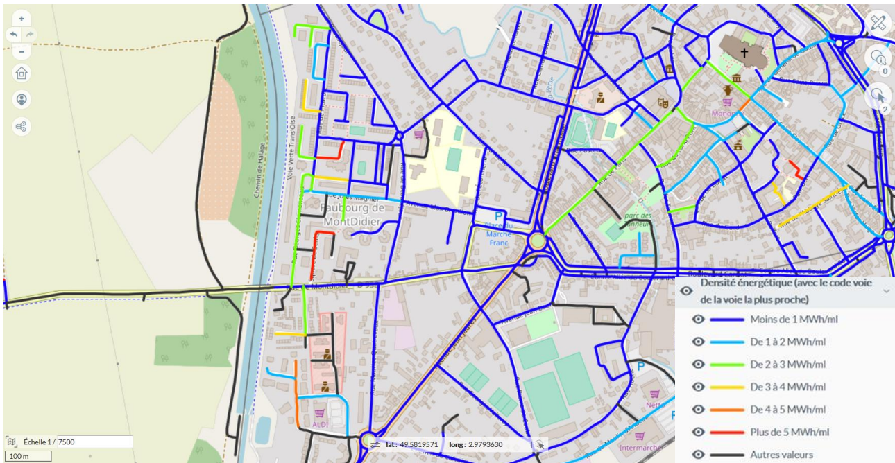
Figure 44 : Potentiel de développement réseaux de chaleur à Noyon quartier Faubourg de MontDidier – Source OPPORTUNITEE BURGEAP
