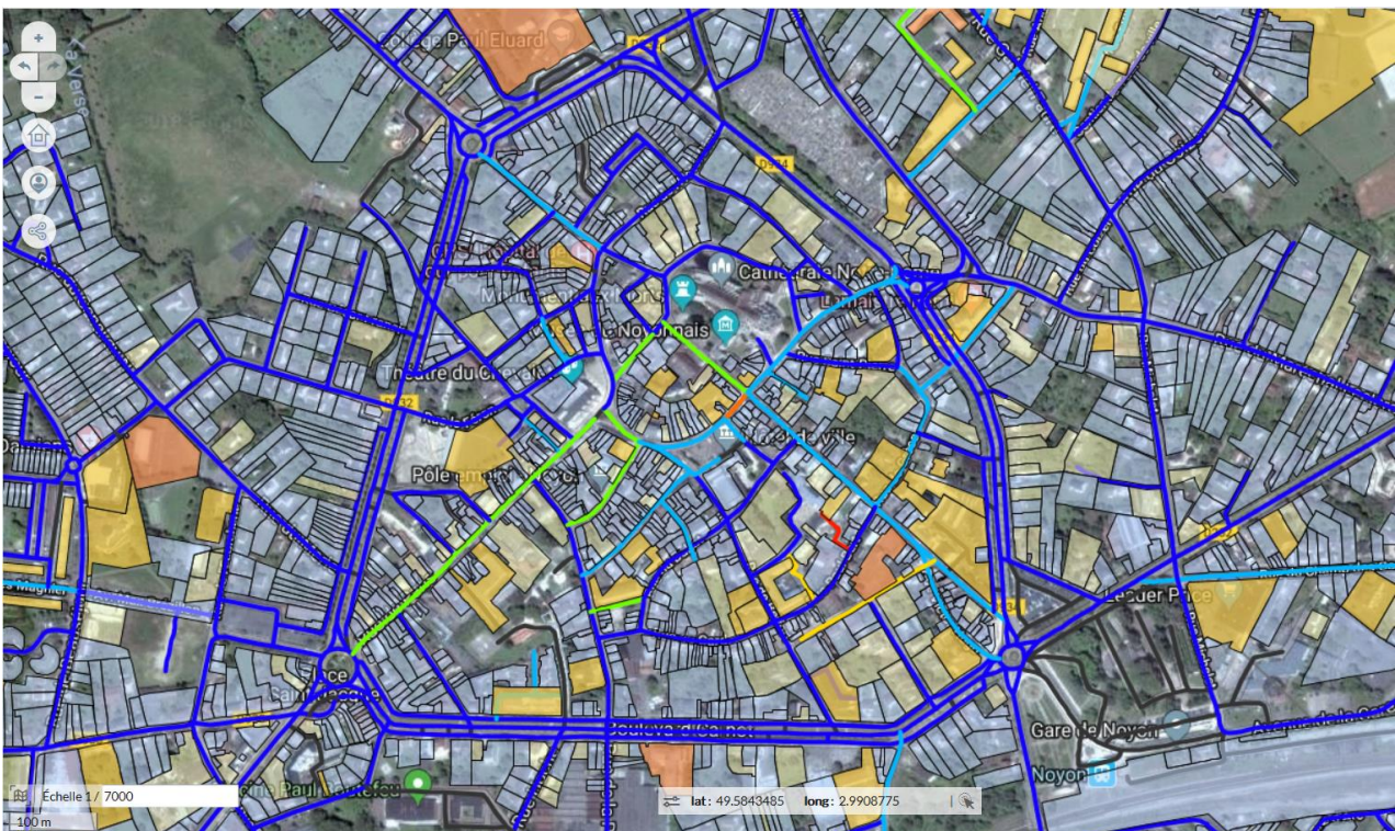
Figure 43 : Potentiel de développement réseaux de chaleur à Noyon centre avec croisement grands consommateurs – Source OPPORTUNITEE BURGEAP
