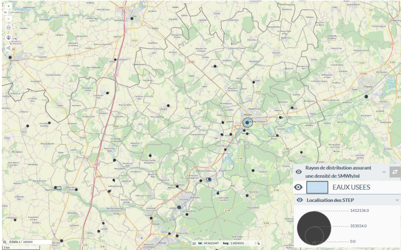
Figure 36 : Gisement de récupération de chaleur sur eaux usées et densité de distribution supérieure à 5 MWh/ml – Source OPPORTUNITE BURGEAP
