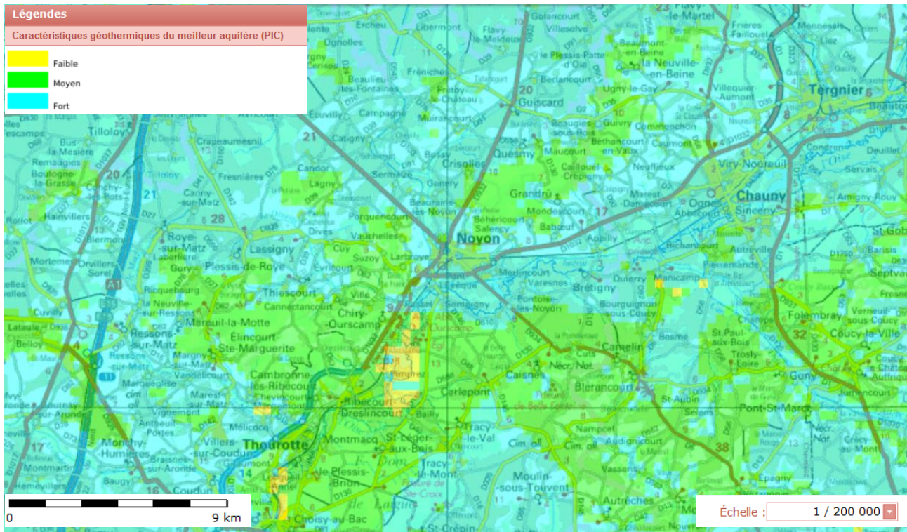
Figure 26 : Gisement géothermique sur aquifère superficiel – Source geothermie-perspectives
