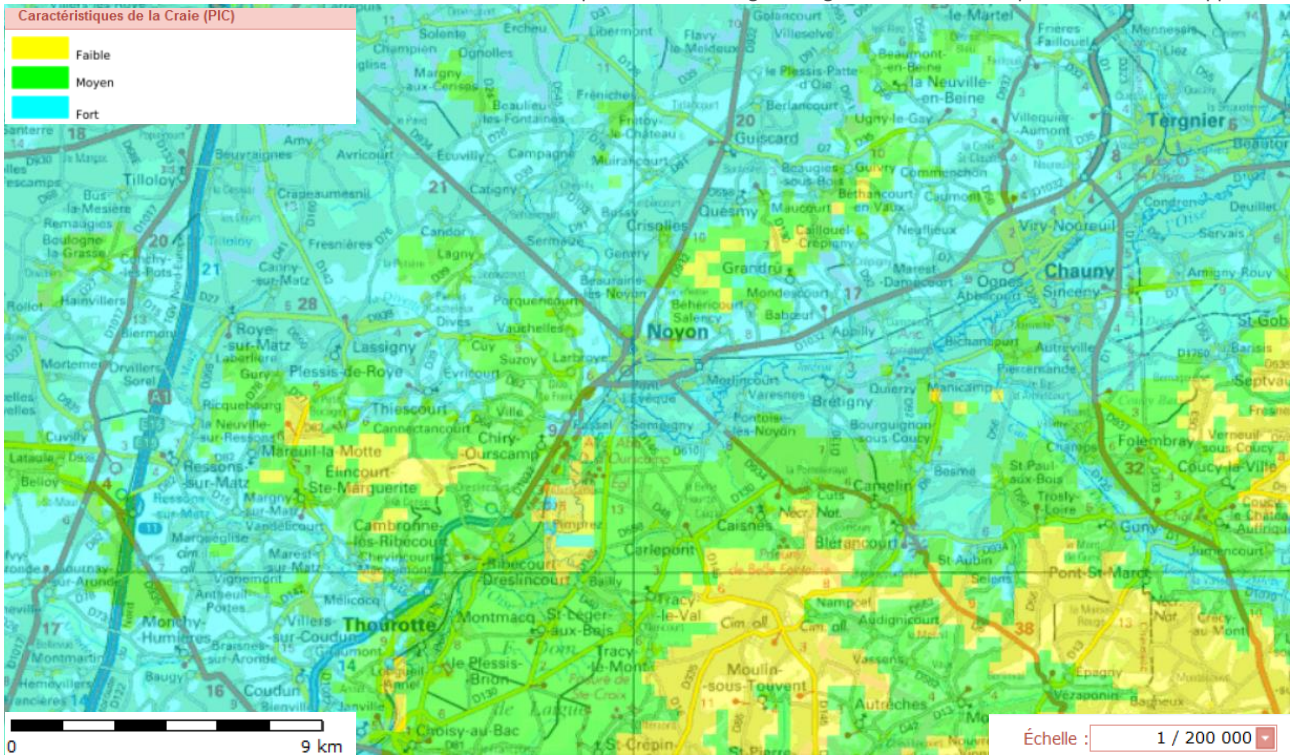
Figure 27 : Gisement géothermique sur aquifère profond (Craie) – Source geothermie-perspectives
