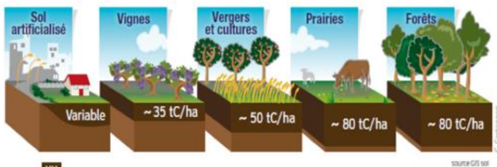
Figure 60 : Schéma des capacité de stockage de carbone selon le type de sol – Source GIS SOL
