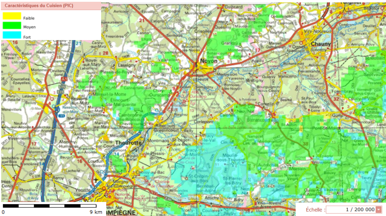
Figure 28 : Gisement géothermique sur aquifère profond (Cuisien) – Source geothermie-perspectives
