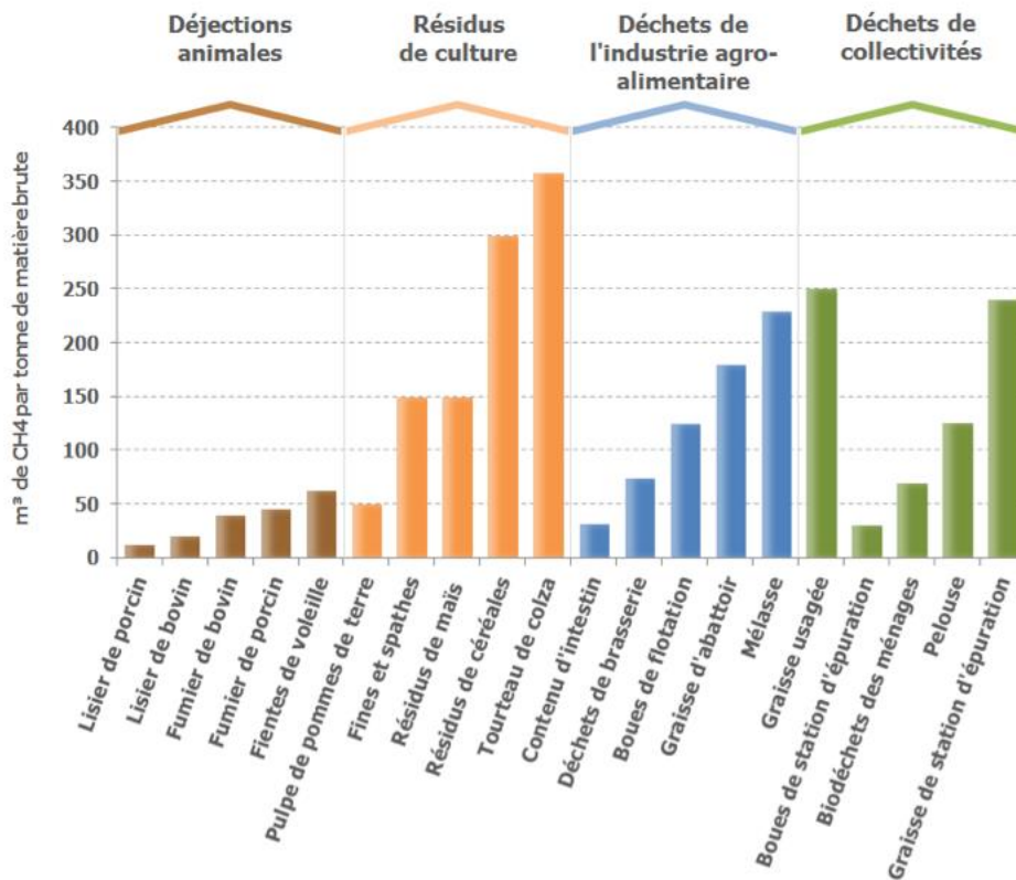
Figure 33 : Pouvoir méthanogène pour les principaux substrats
