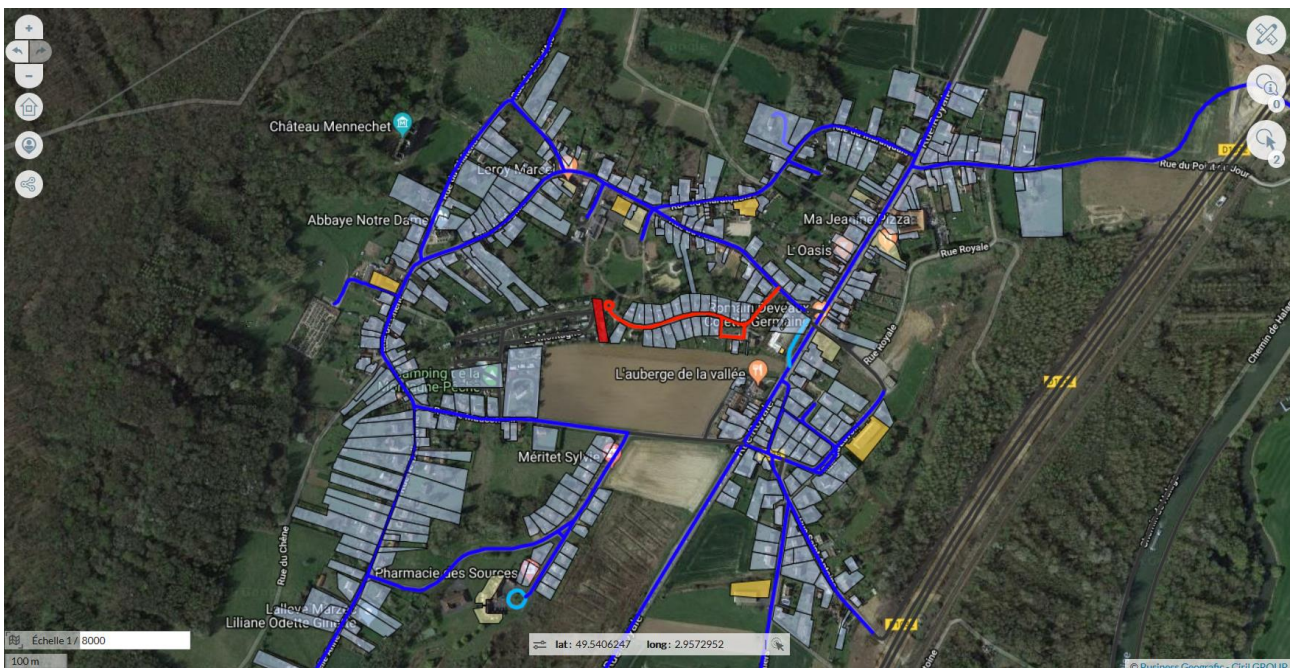
Figure 51 : Raccordements possibles de gros consommateurs à Chiry-Ourscamp – Source OPPORTUNITEE BURGEAP
